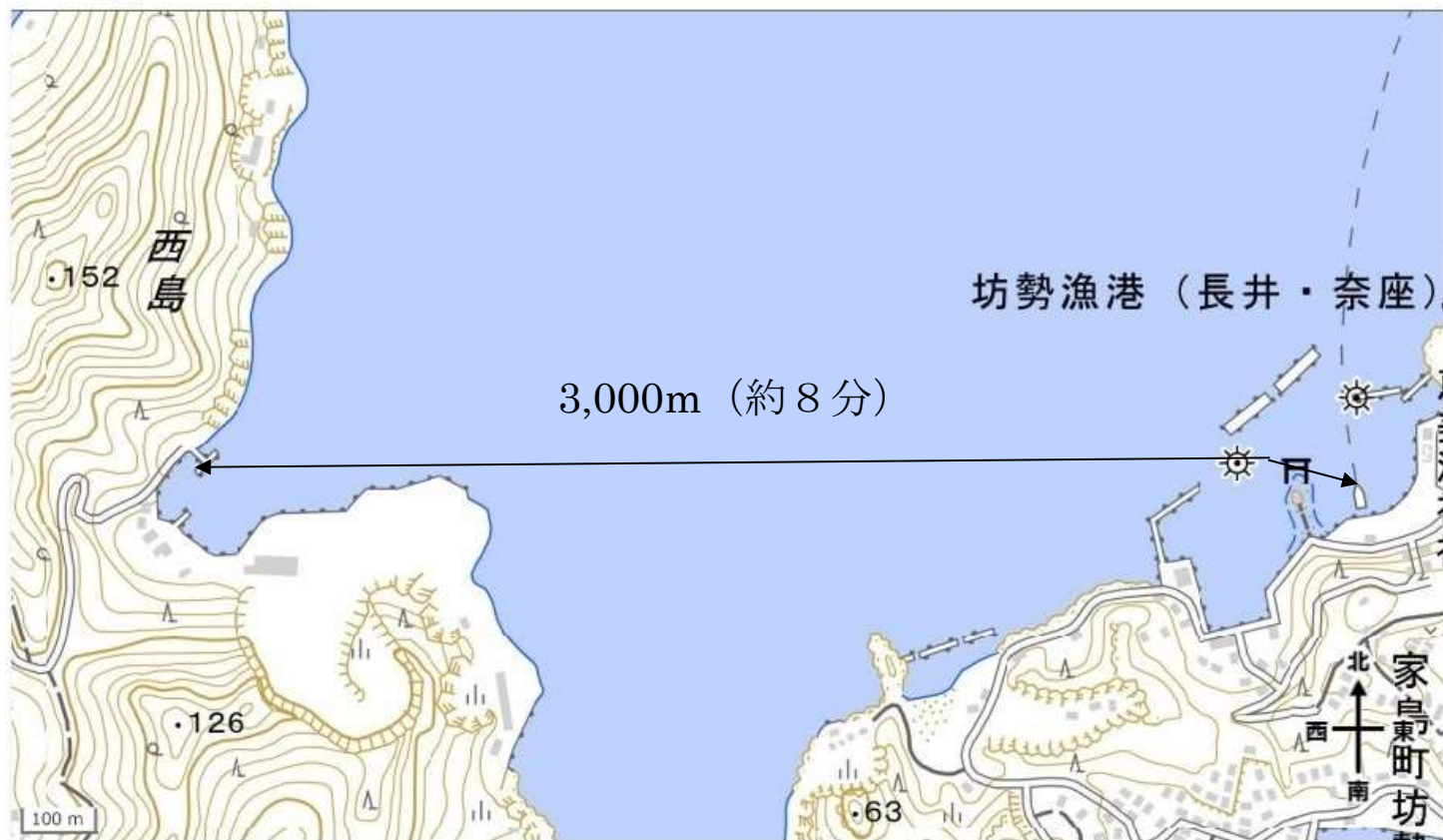
運航基準図
